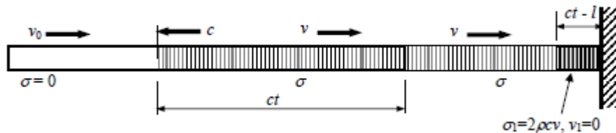
Figura A.9 – riflessione in corrispondenza di una estremità fissa (dopo la riflessione)
