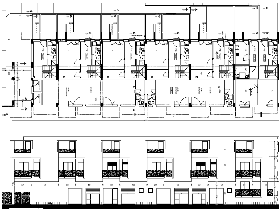
Fig. 5.29 – Pianta del piano terra e prospetto ovest del progetto degli alloggi a schiera su piazza S. Maria delle Salette (Comune di Catania)
