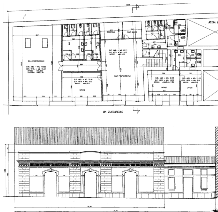
Fig. 5.30 – Pianta del piano terra e prospetto principale del progetto di rifunzionalizzazione dell'ex cinema Midulla in via Belfiore (Comune di Catania)
