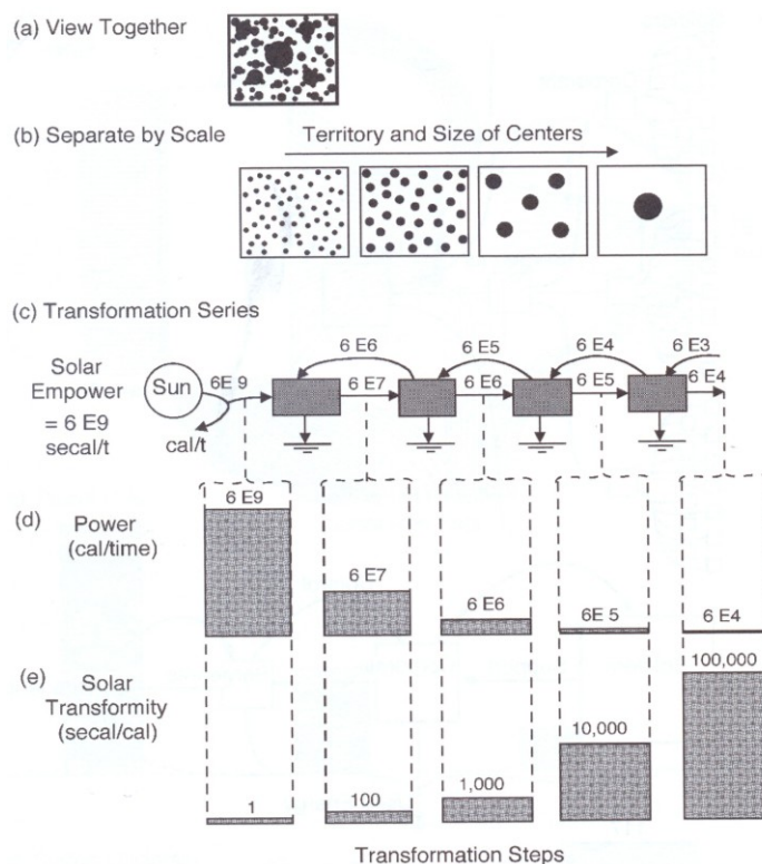
Fig. 2.10 – Trasferimenti energetici in un ecosistema (Odum H. T., 2007)
