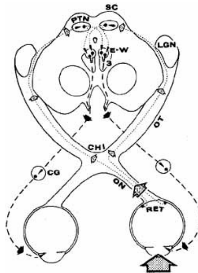
Figura 1 Innervazione delle fibre parasimpatiche che originano nel nucleo di Westphal subnucleus (EW) . Gli assoni parasimpatici entrano nell'orbita come parte della branca inferiore del nervo oculomotore. Le fibre (pre)gangliari prendono contatto sinaptico a livello del ganglio ciliare prima di innervare il muscolo costrittore della pupilla. (SC, superior colliculus; PTN, pretectal nucleus; LGN, lateral geniculate; OT, optic tract; CHI, chiasm; ON, optic nerve; RET, retina).
