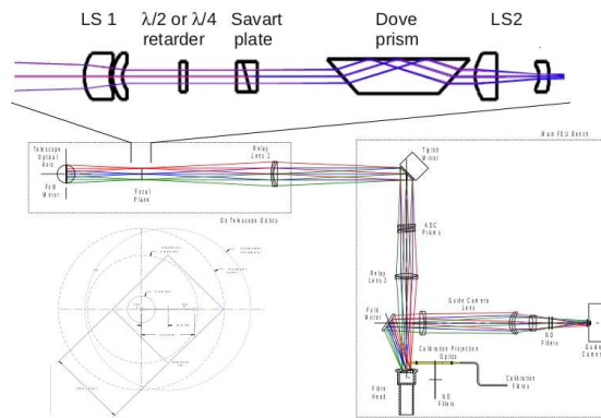
Figure 2. Optical scheme of the polarimeter. Sostituire con nuova figura
