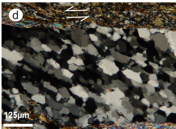
Fig. 10 - Microstrutture prodotte dall'evento deformativo di taglio ( D_1 ) in orto e paraderivati indicanti un senso di taglio sinistro: (a) mica chiara con tessitura tipo fish in leucogneiss; (b) indicatore cinematico da transazionale a \delta -type in paragneiss; (c) porfiroclasto di plagioclasio tipo \sigma in gneiss leucocratico; (d) oblique foliation in paraderivato; (e) plagioclasio con struttura domino-type in leucogneiss.
