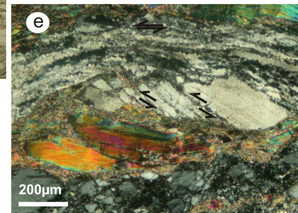
Fig. 10 - Microstrutture prodotte dall'evento deformativo di taglio ( D_1 ) in orto e paraderivati indicanti un senso di taglio sinistro: (a) mica chiara con tessitura tipo fish in leucogneiss; (b) indicatore cinematico da transazionale a \delta -type in paragneiss; (c) porfiroclasto di plagioclasio tipo \sigma in gneiss leucocratico; (d) oblique foliation in paraderivato; (e) plagioclasio con struttura domino-type in leucogneiss.
