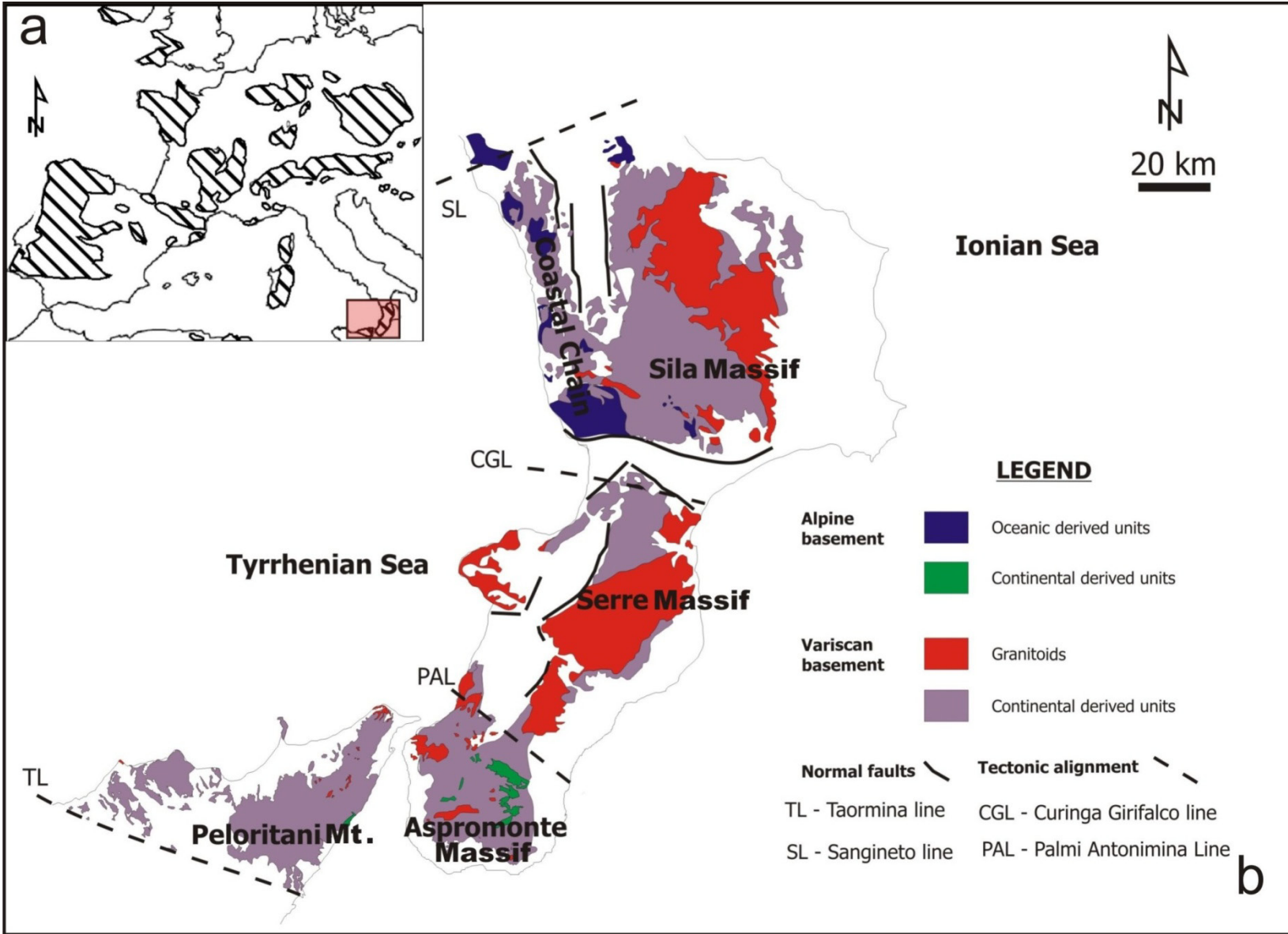
Fig.1: a) Ubicazione dei basamenti cristallini ercinici relitti nel settore occidentale del bacino mediterraneo (da von Raumer, 2002); b) Carta geologica schematica del basamento cristallino Calabro-Peloritano (da Angi et al., 2010)
